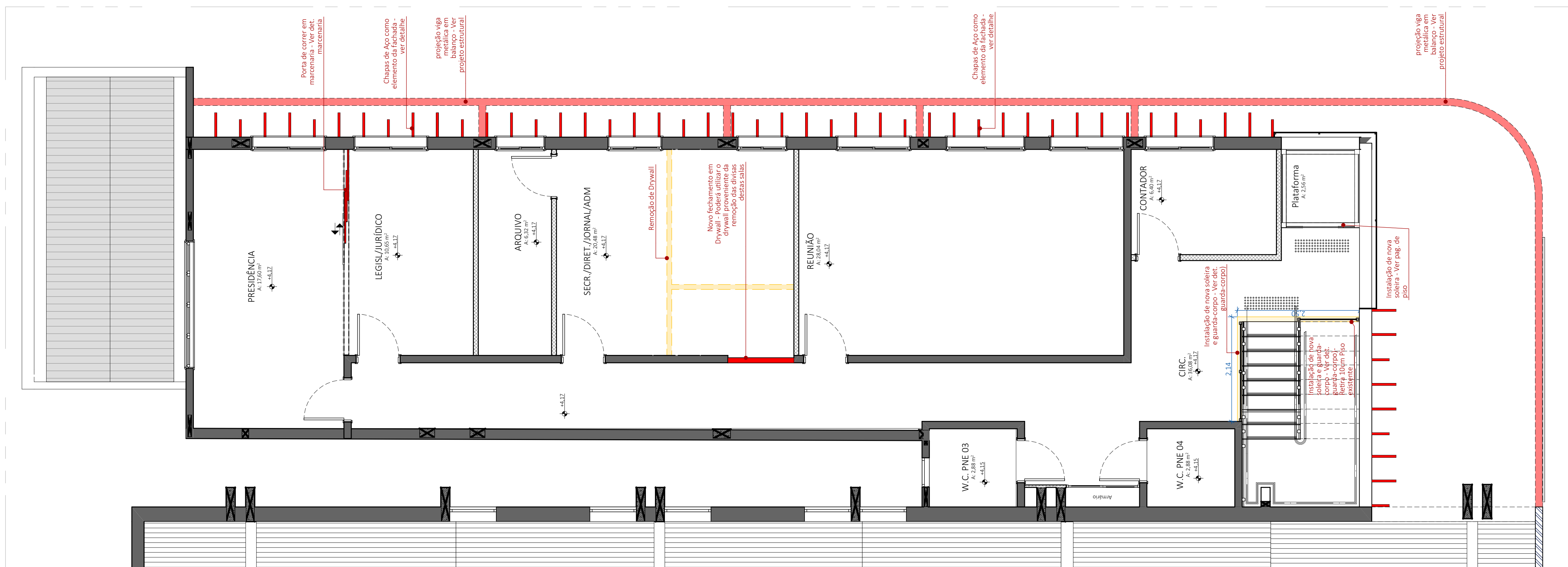
1º PAV - DEMOLIÇÃO E CONSTRUÇÃO Esc.:1:50
