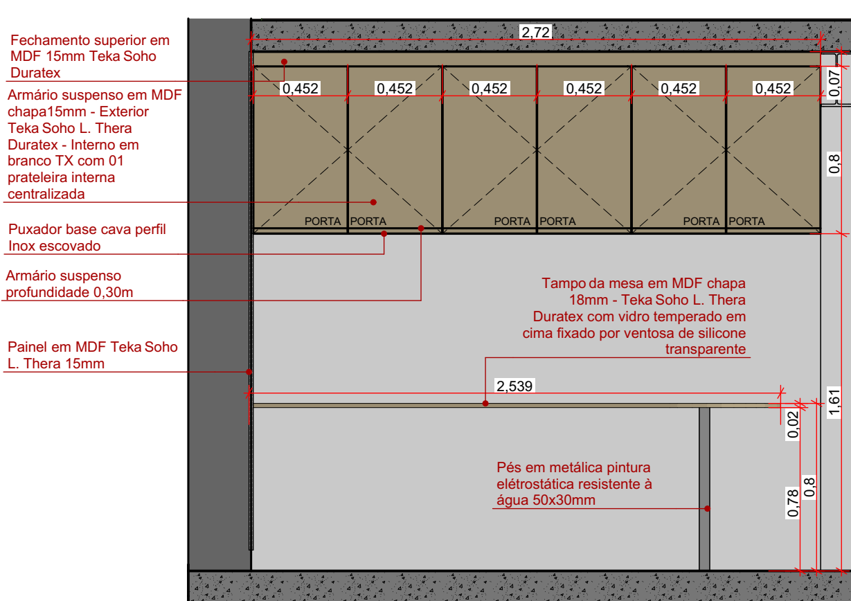
COZINHA - Elev. 03 ESC: 1:25
