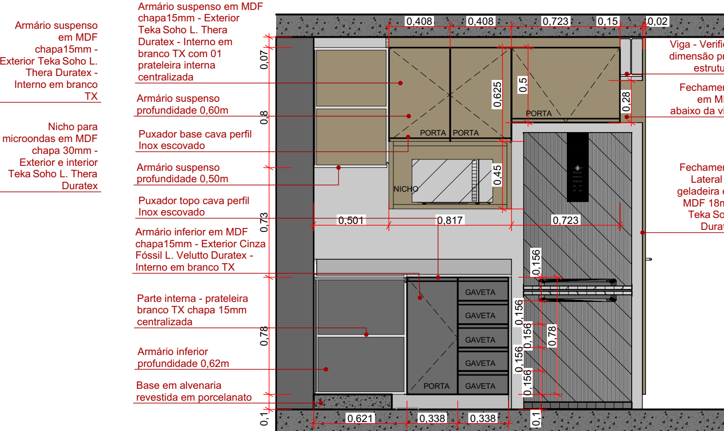
COZINHA - Elev. 02 ESC: 1:25
