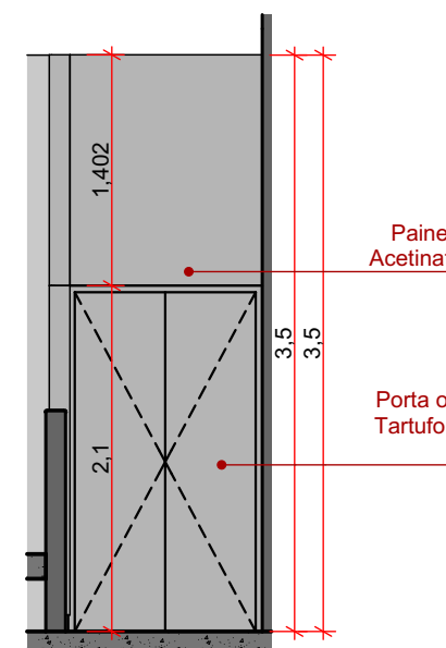
PAINEL E PORTA - ELEV. 03 ESC: 1:50
