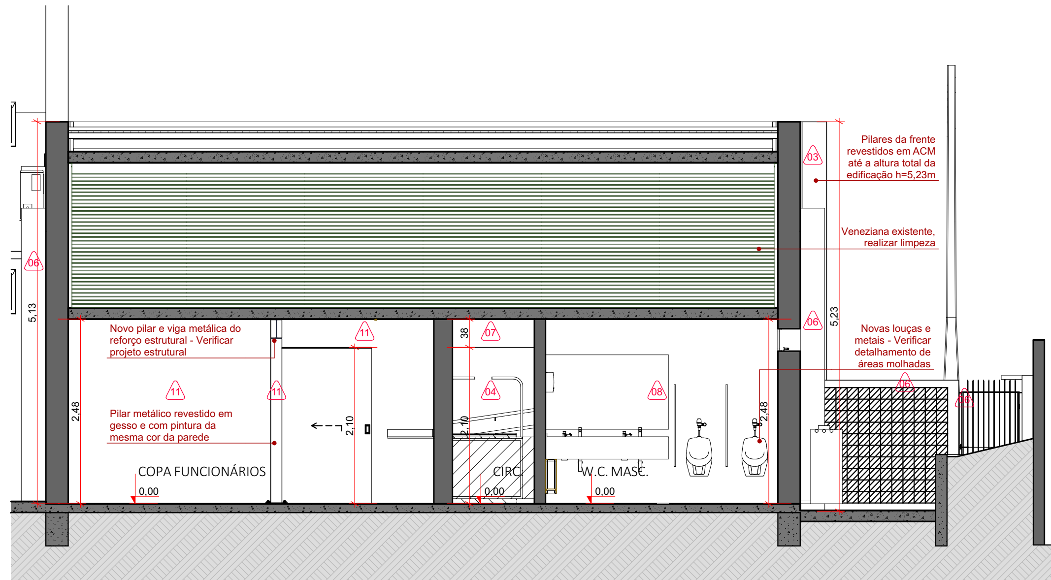
CORTE D-D ESC: 1:50
