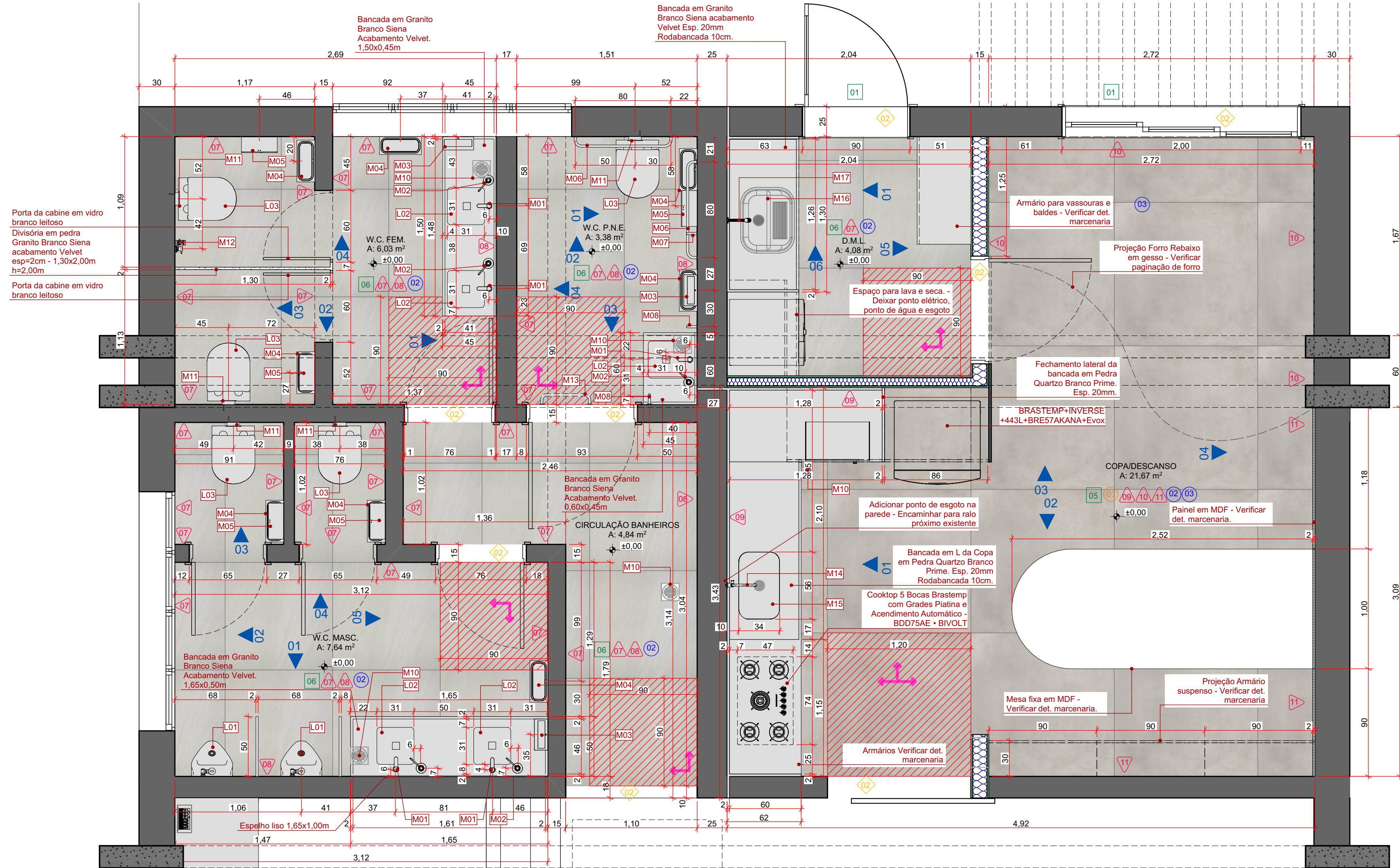
PAINTA BAIXA - ÁREAS MOLHADAS ESC: 1:25
