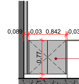
PORTINHOLA - Elev. 07 ESC: 1:50
