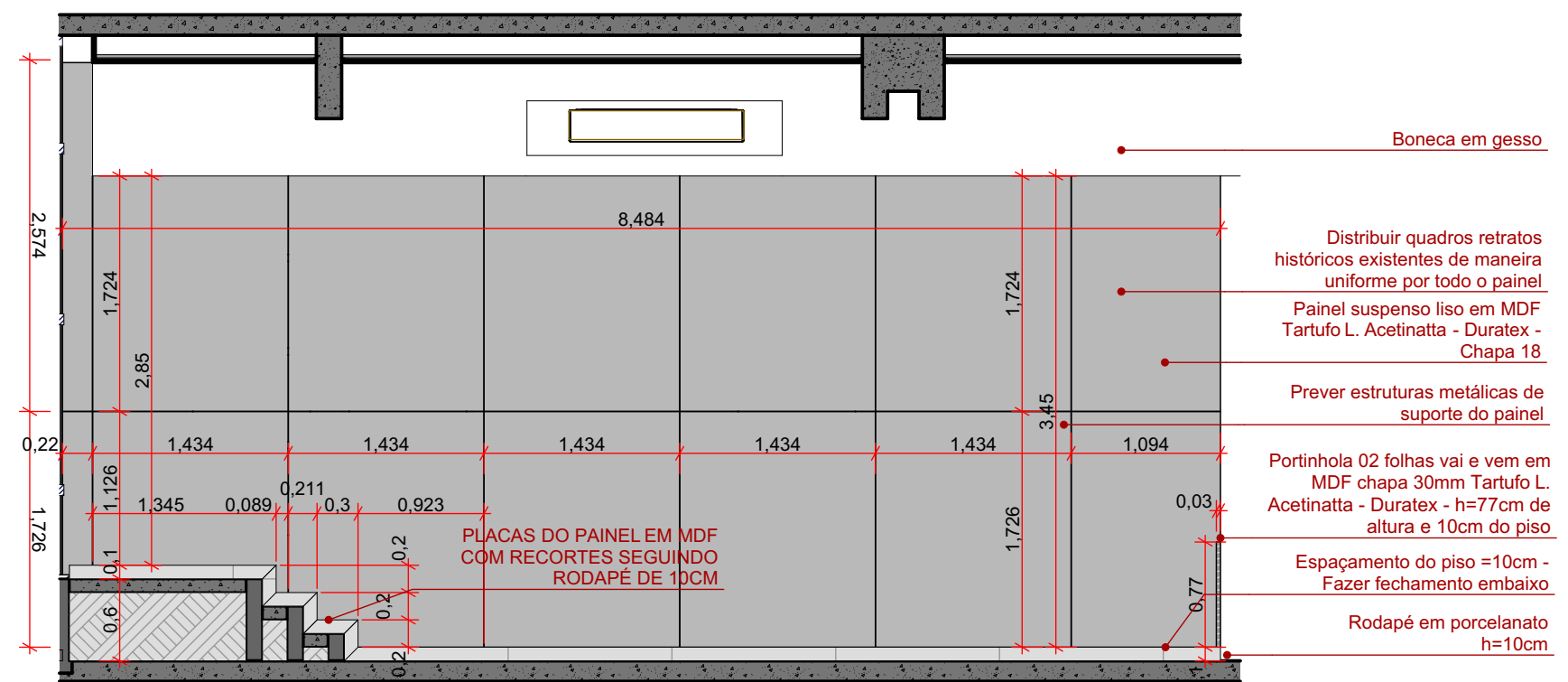
PAINEL - ELEV. 02 ESC: 1:50
