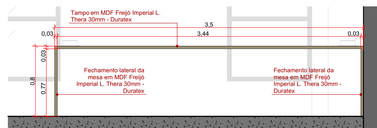
MESA DE APOIO - ELEV. 06 ESC: 1:25
