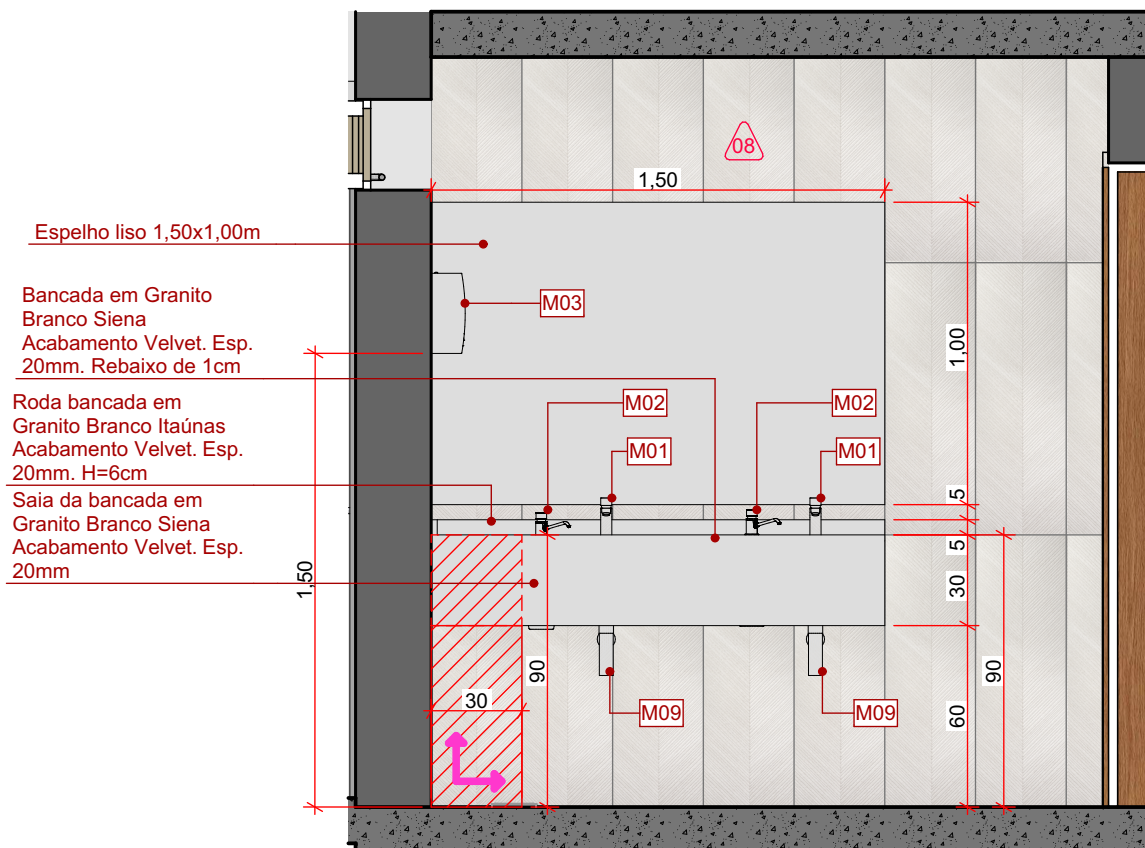
W.C. FEM - Elev. 01 ESC: 1:25
