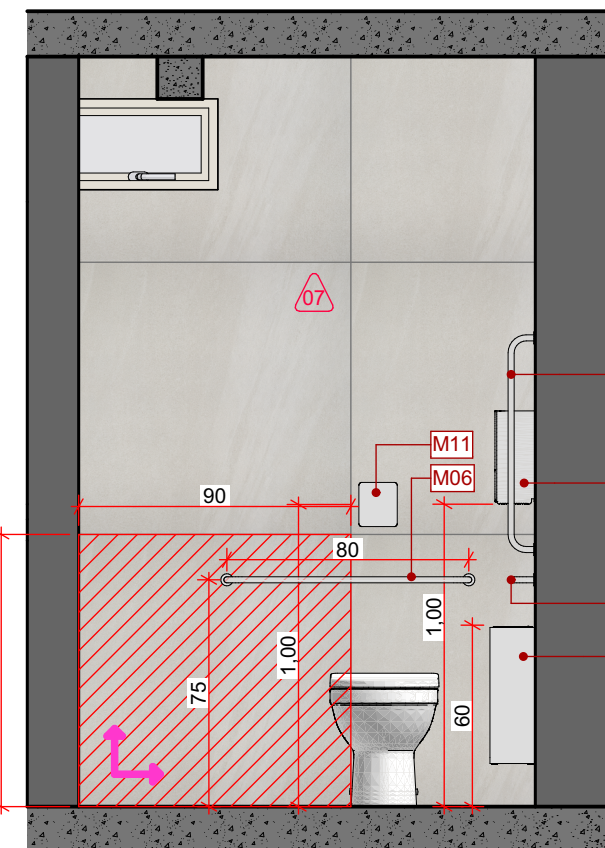
W.C. PNE - Elev. 01 ESC: 1:25
