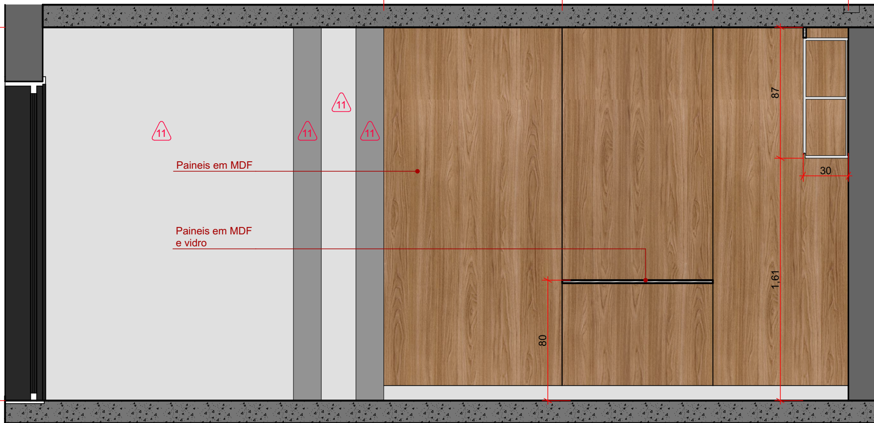
COPA / DESCANSO - Elev. 04 ESC: 1:25
