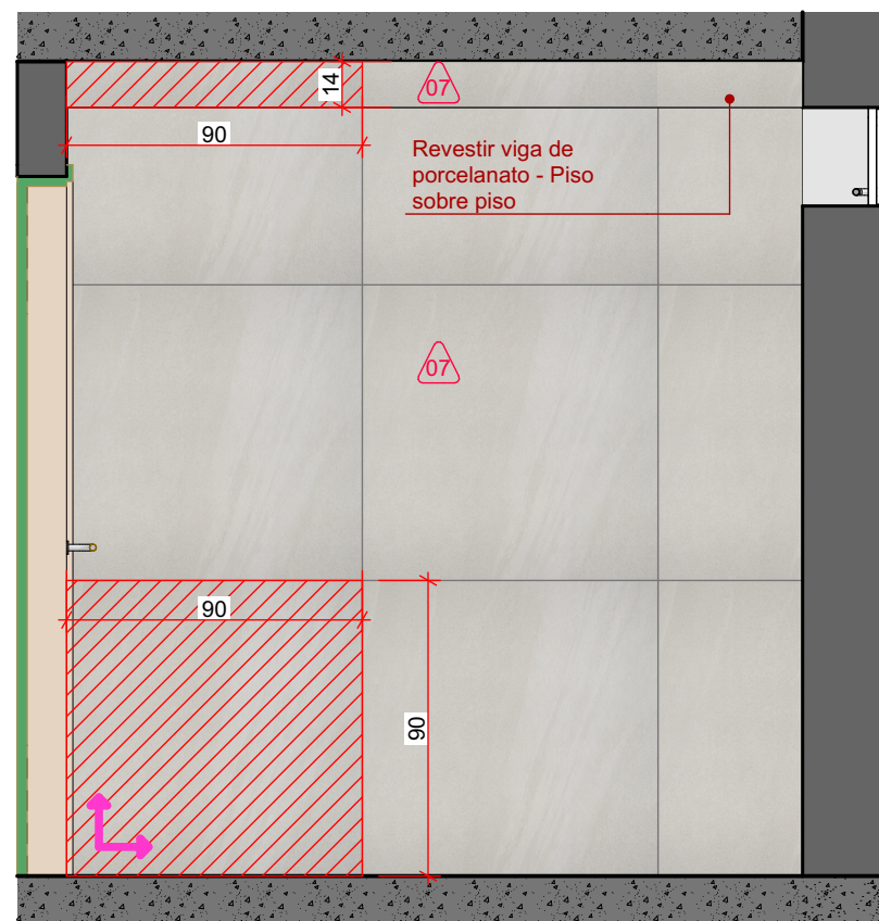
W.C. PNE - Elev. 04 ESC: 1:25
