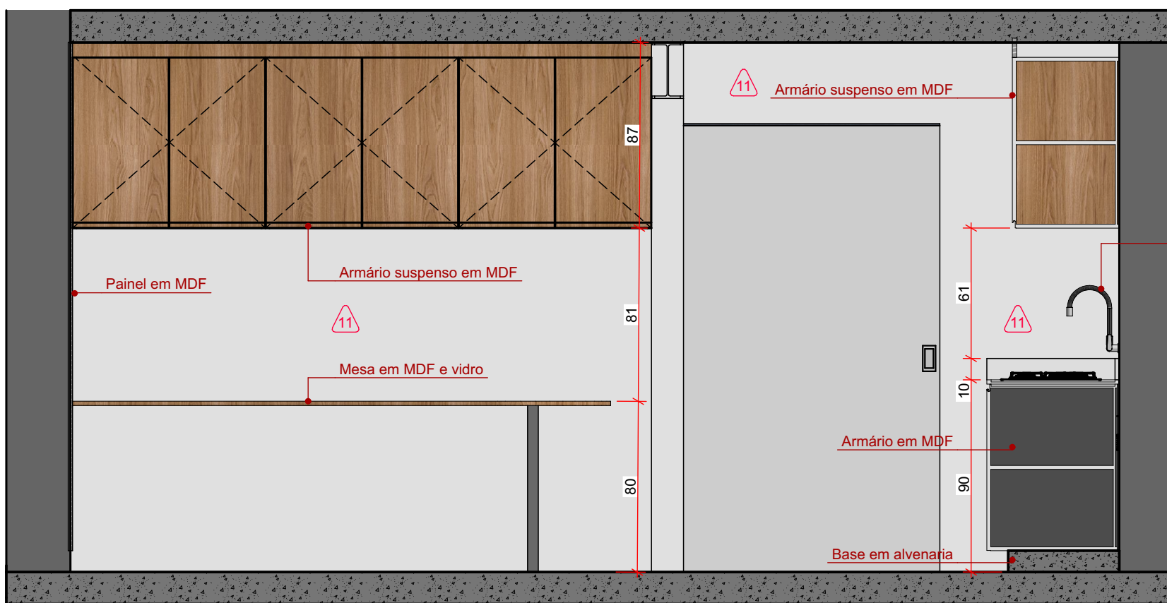
COPA - Elev. 02 ESC: 1:25
