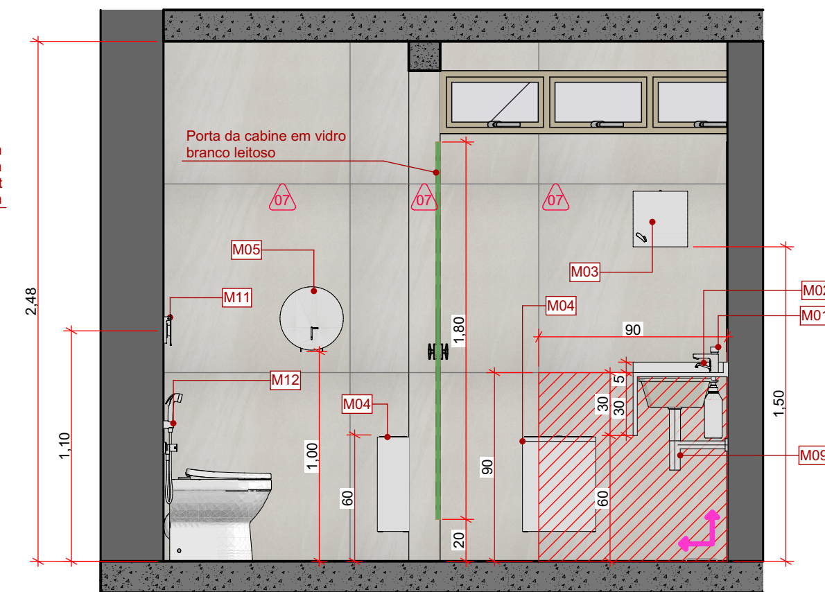
W.C. FEM - Elev. 04 ESC: 1:25
