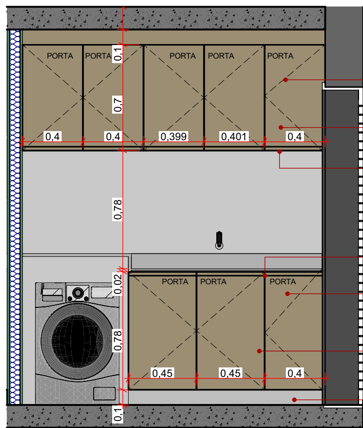
D.M.L. - Elev. 01 ESC: 1:25
