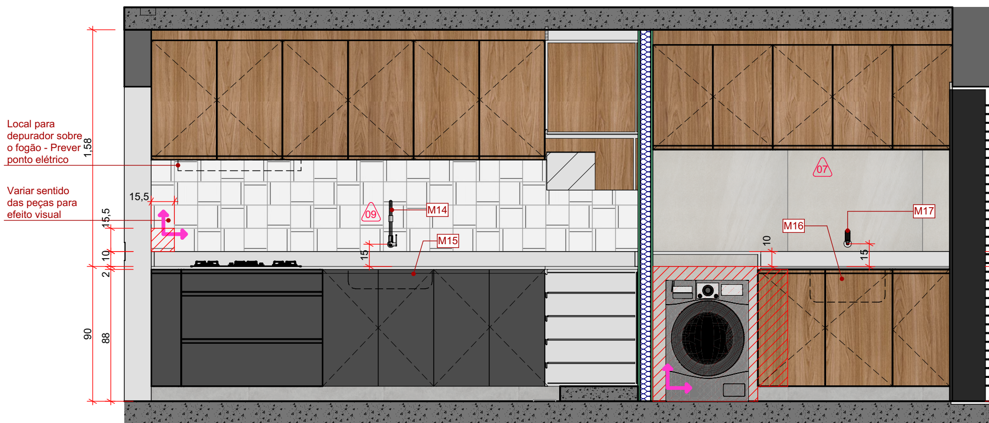
COPA / DML - Elev. 01 ESC: 1:25
