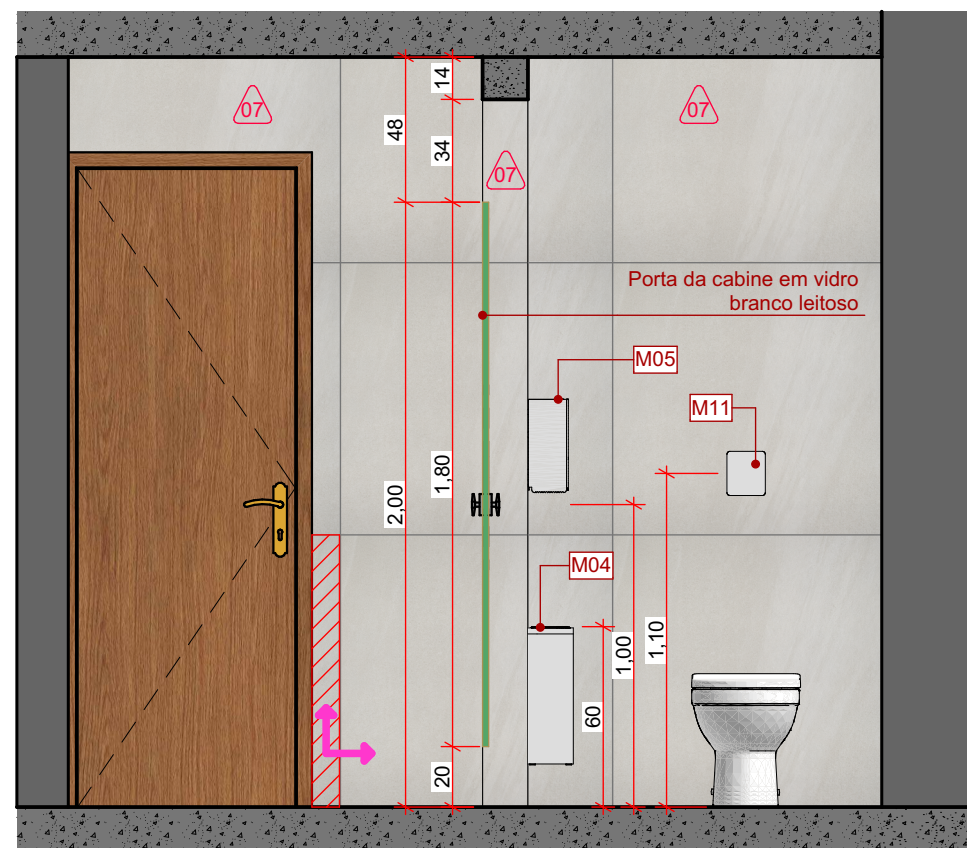
W.C. FEM - Elev. 02 ESC: 1:25
