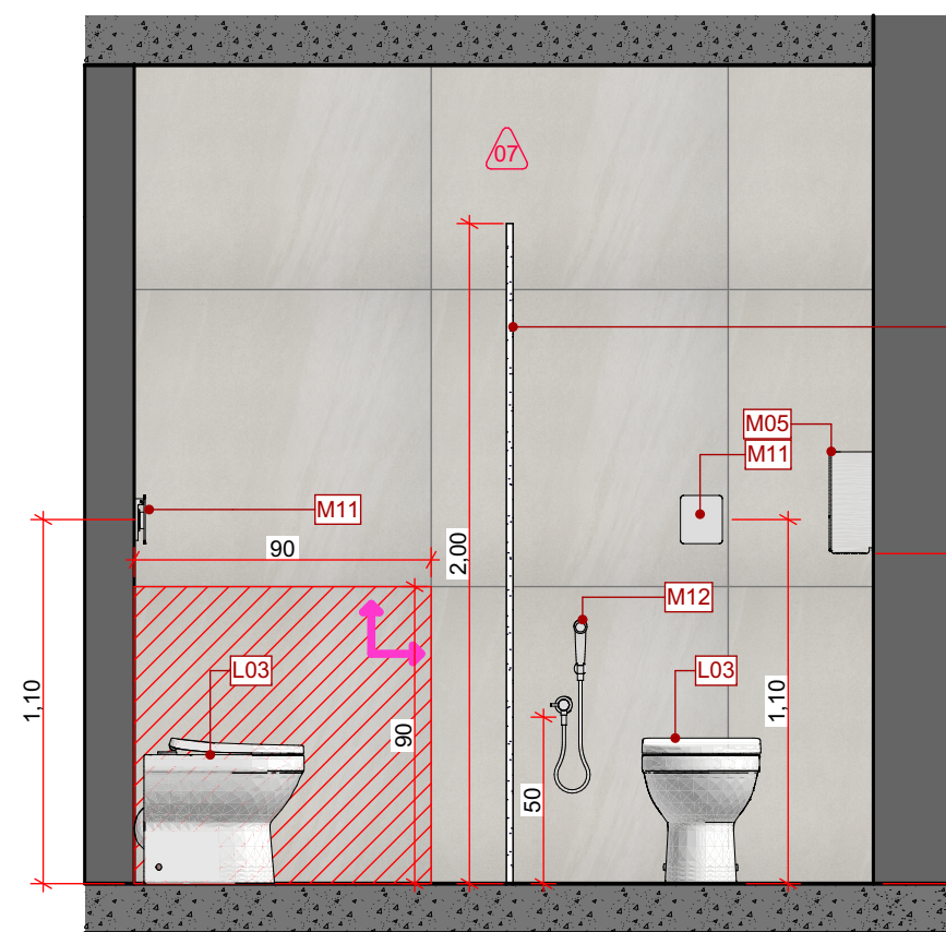
W.C. FEM - Elev. 03 ESC: 1:25
