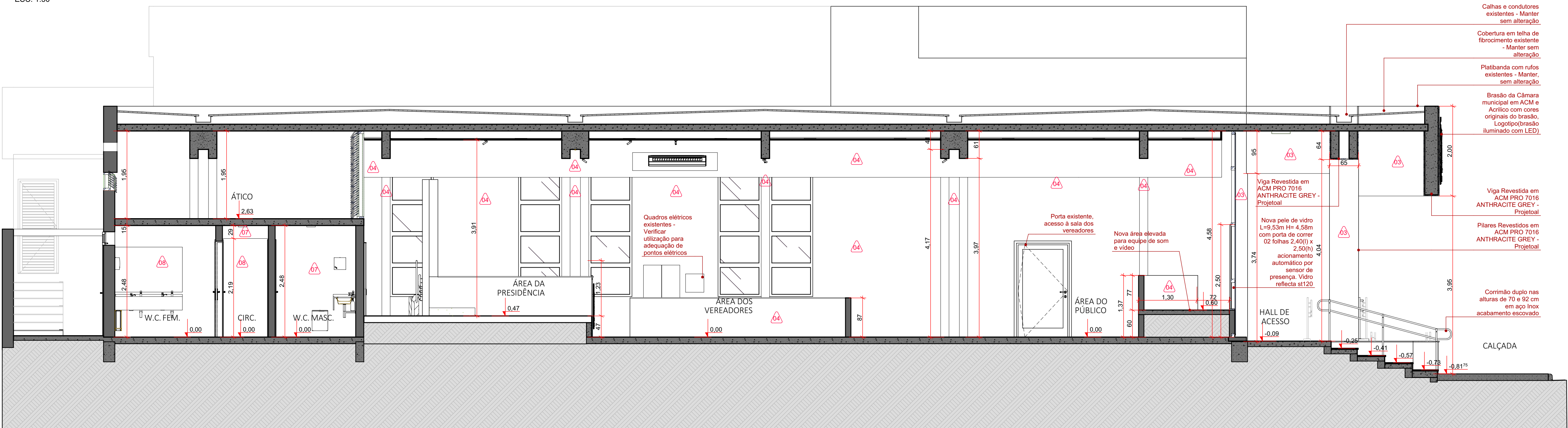
CORTE C-C ESC: 1:50
