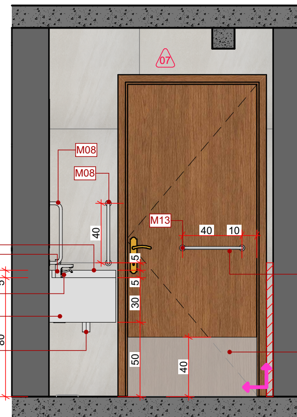
W.C. PNE - Elev. 03 ESC: 1:25
