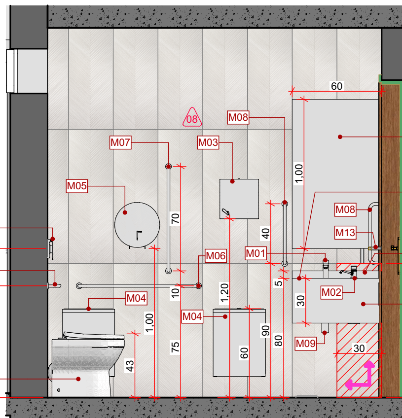
W.C. PNE - Elev. 01 ESC: 1:25
