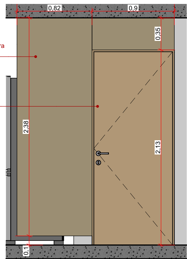
COZINHA - Elev. 05 ESC: 1:25
