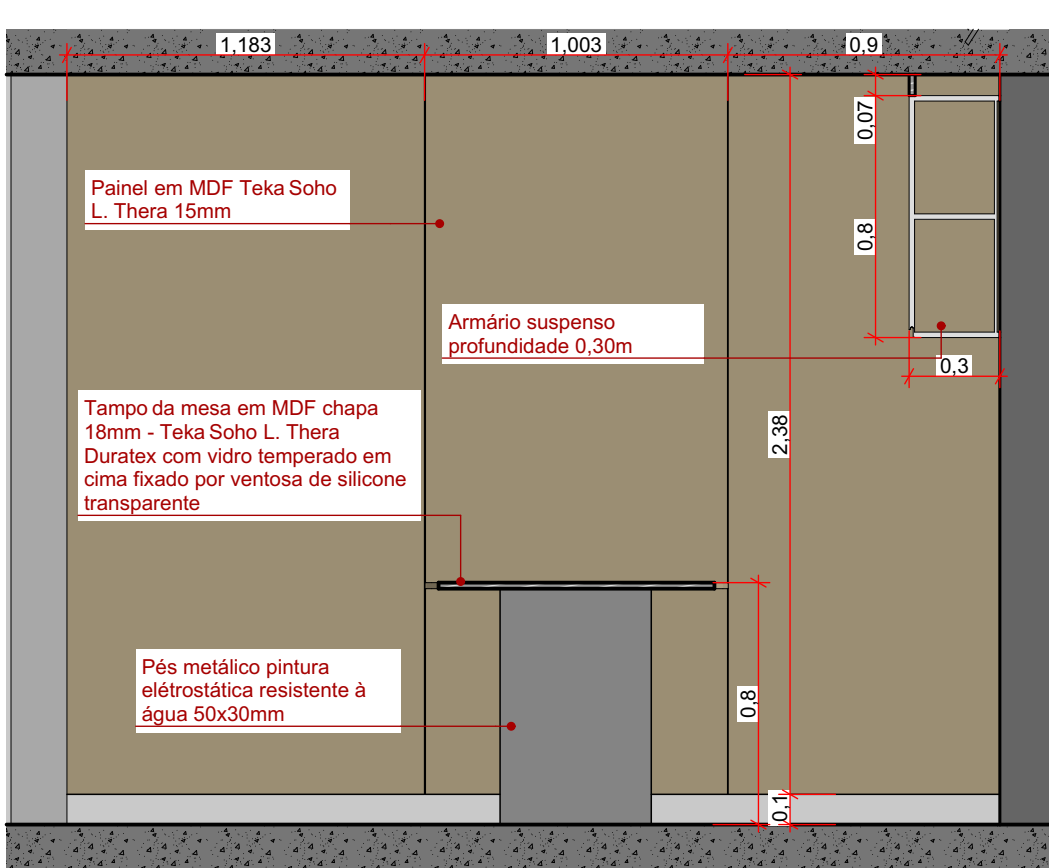
PAINEL E PORTA - ELEV. 03 ESC: 1:50
