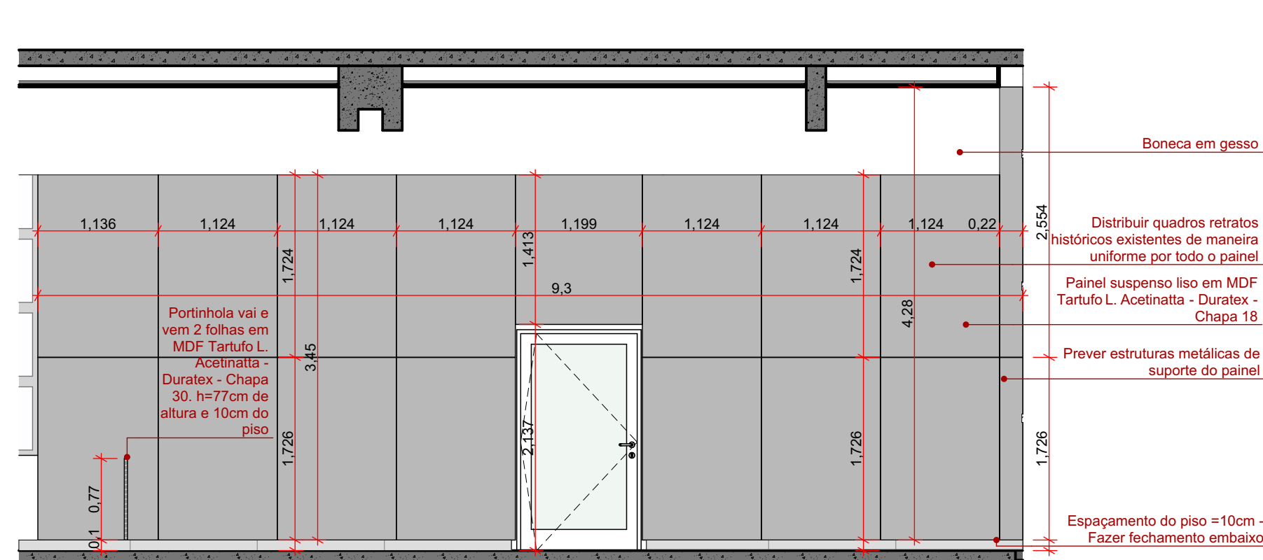
PAINEL - ELEV. 01 ESC: 1:50
