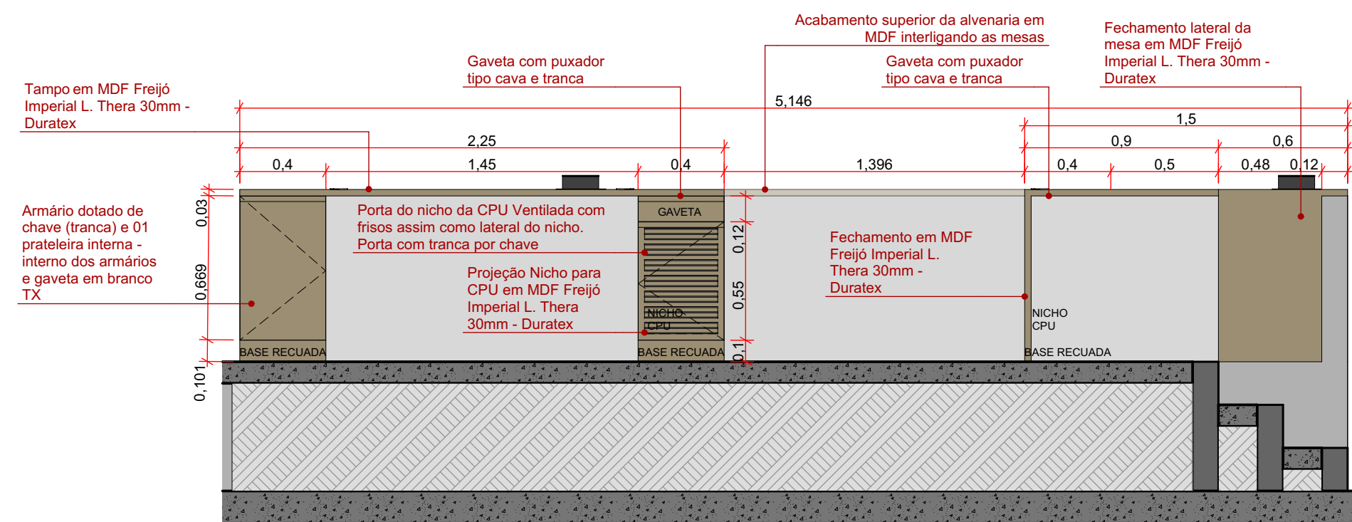
MESA DE SOM E VÍDEO - Elev. 04 ESC: 1:25
