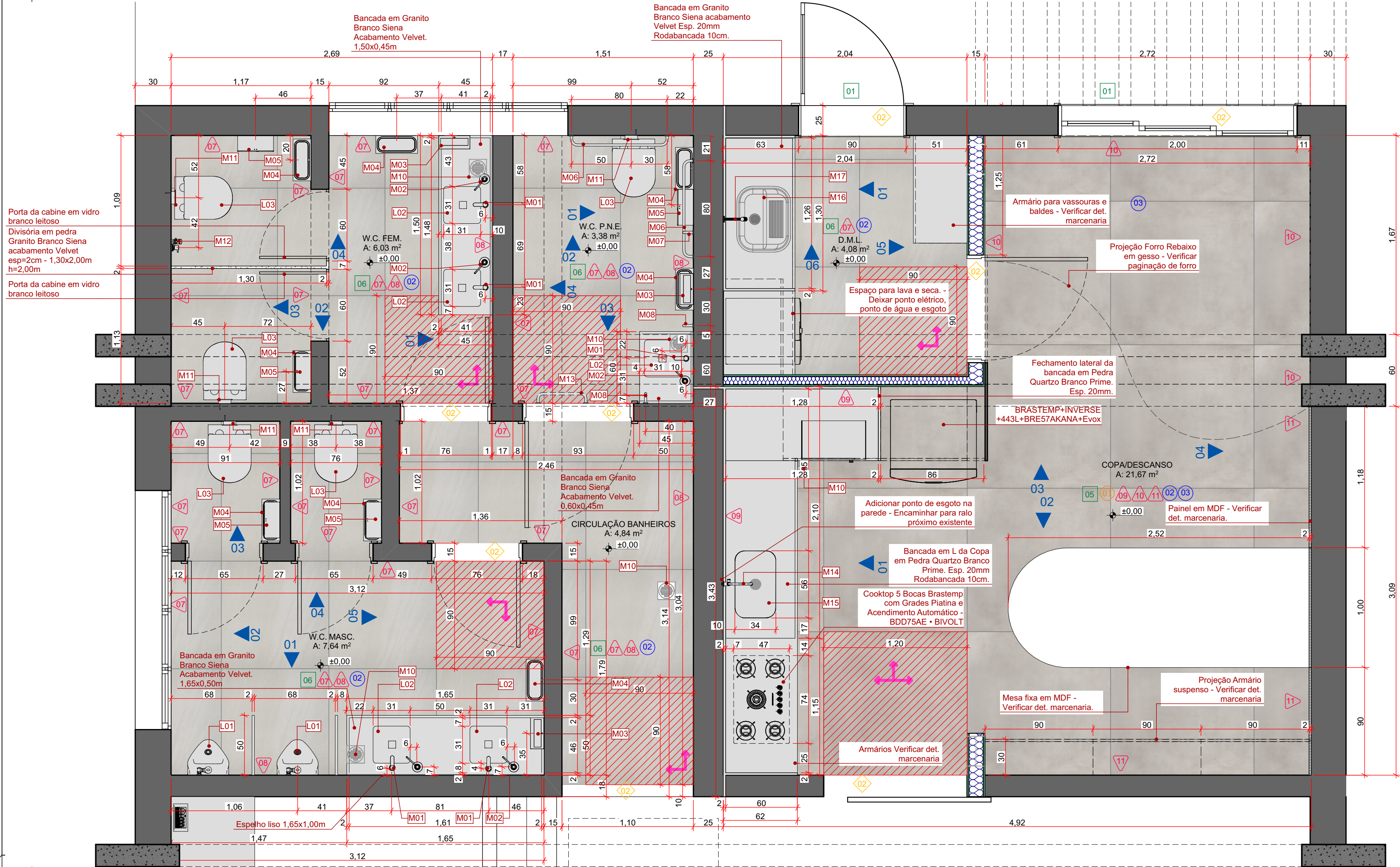
PLANTA BAIXA - ÁREAS MOLHADAS ESC: 1:25
