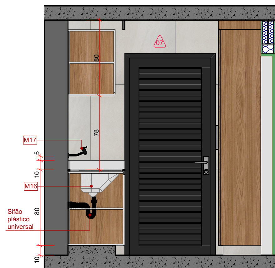
D.M.L. - Elev. 06 ESC: 1:25
