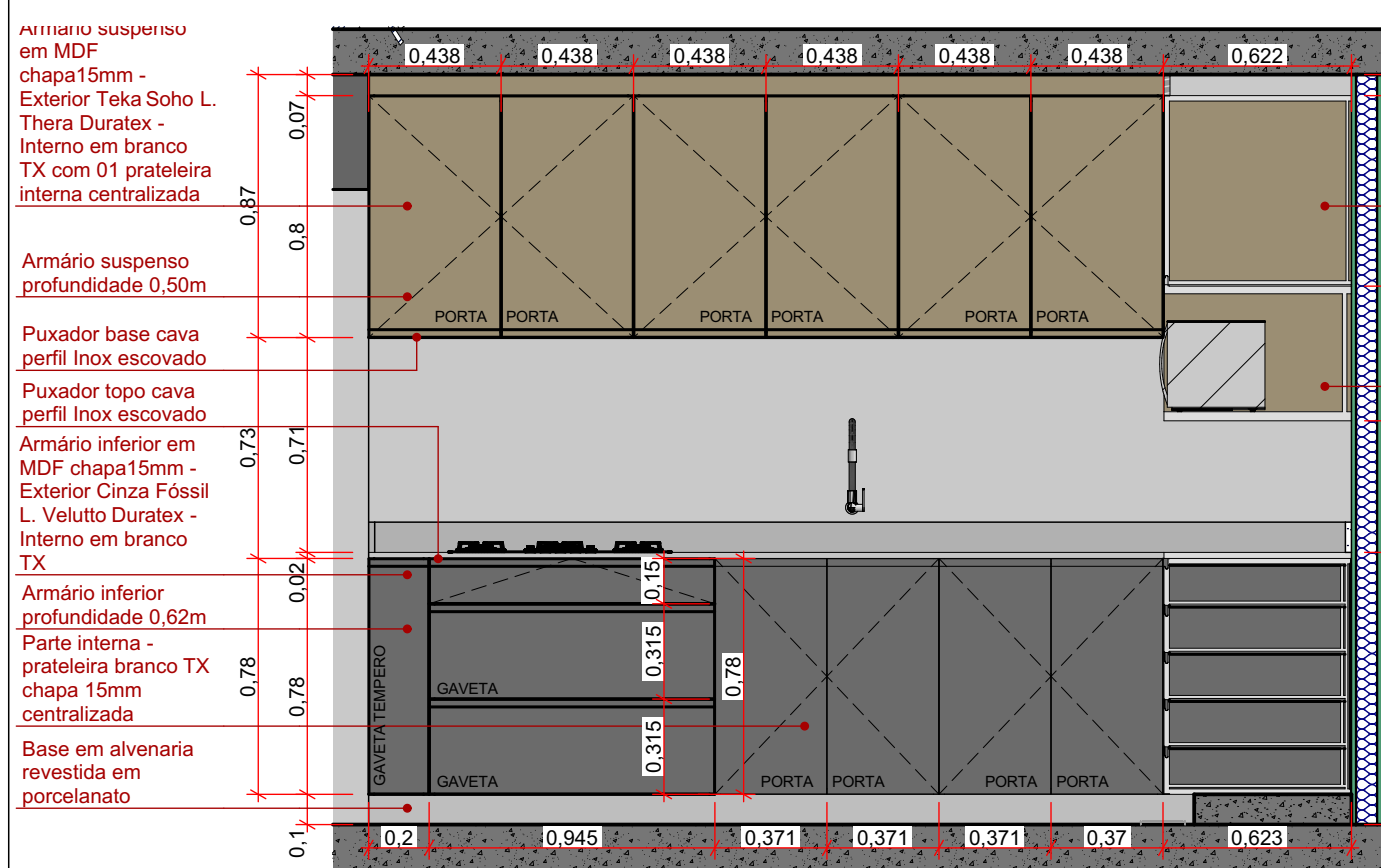
COZINHA - Elev. 01 ESC: 1:25
