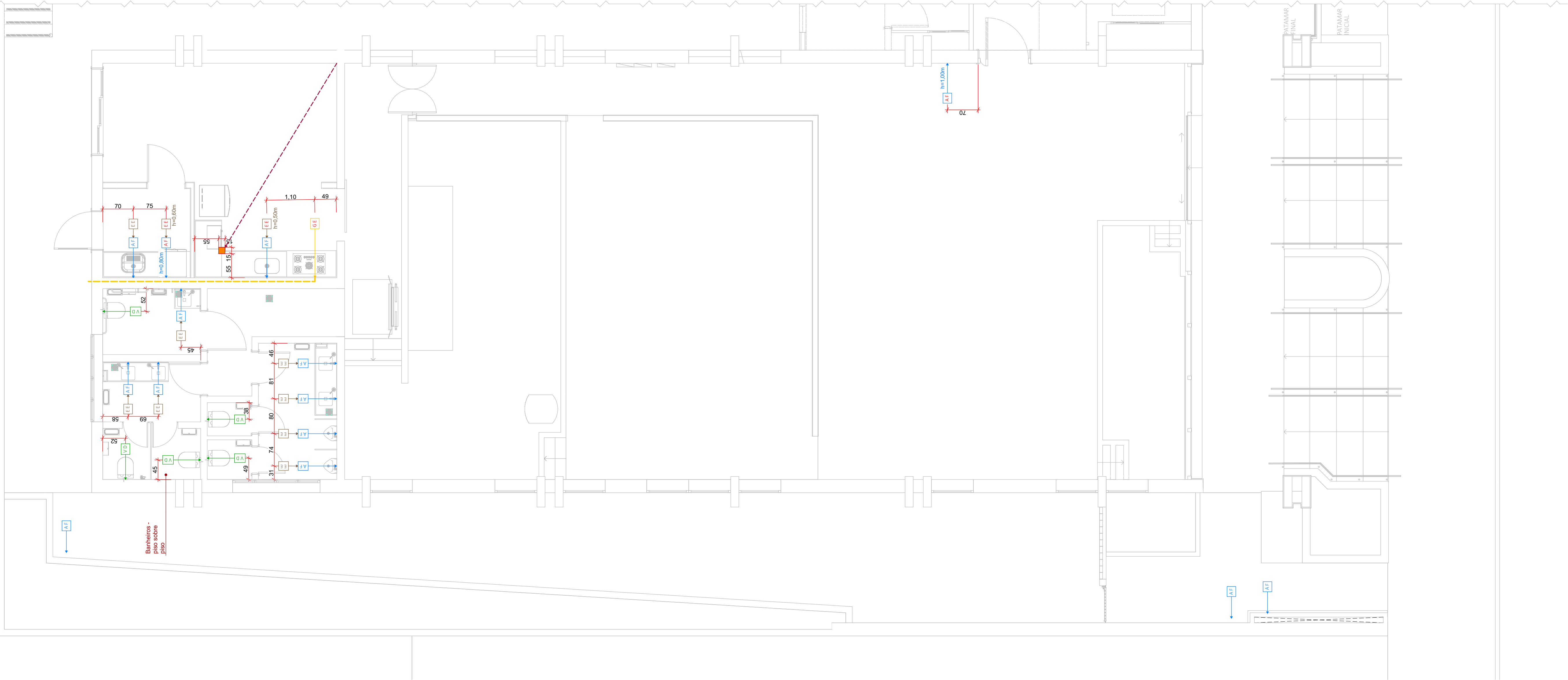
PONTOS HIDRÁULICOS E ESGOTO - TÉRREO 1:50
