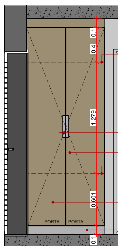
D.M.L. - Elev. 02 ESC: 1:25
